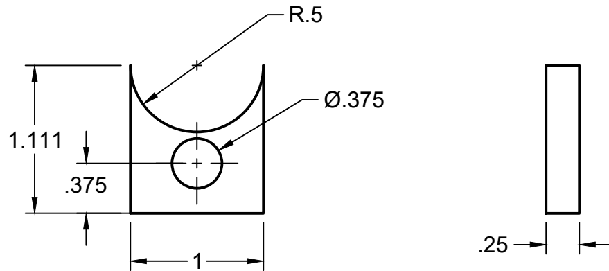
ITEM 15 - RIGHT GUIDE EXTENSION
