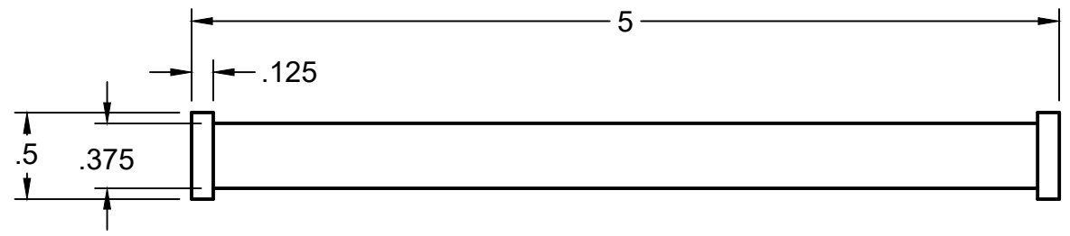
ITEM 3 - HANDLE
