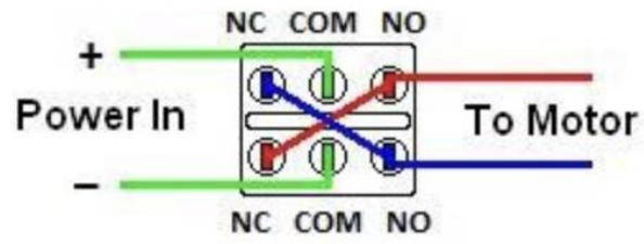
Figure 1: Le circuit entre le commutateur et la source d'électricité et l'actionneur linéaire
